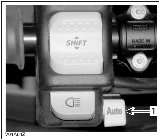
1. Manual/autoshift selector
